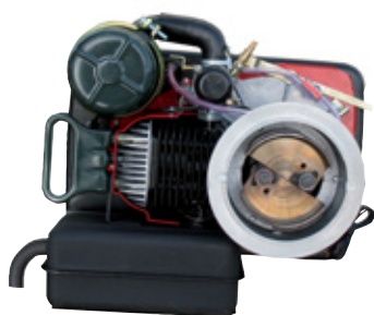
Odstředivá spojka Ø 120 mm
