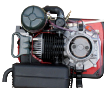
Odstředivá spojka Ø 80 mm
